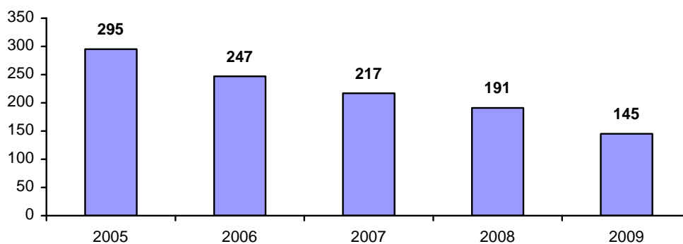
Figura 4. Infracțiuni săvârșite de minori la 100 mii populație în vârstă de 0-17 ani
